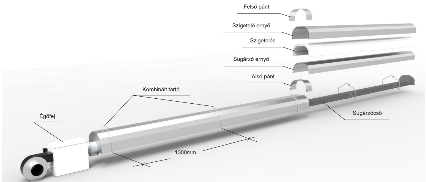
2. ábra: Az egyenes kivitelű készülék felépítése
