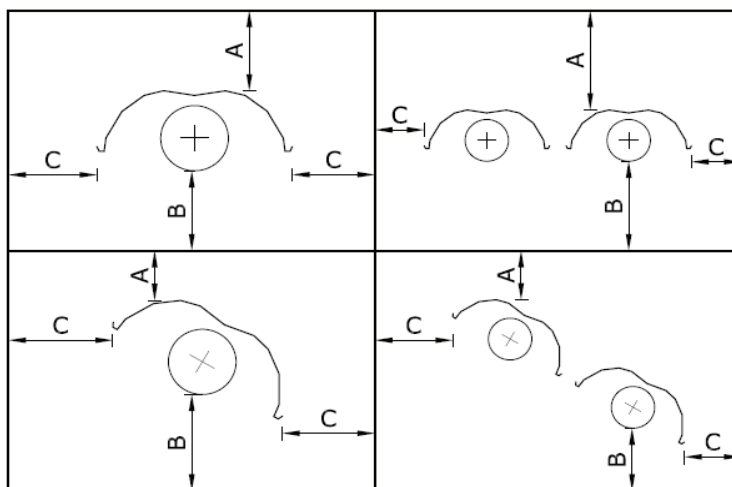
20. ábra: Tűzvédelmi távolságok
