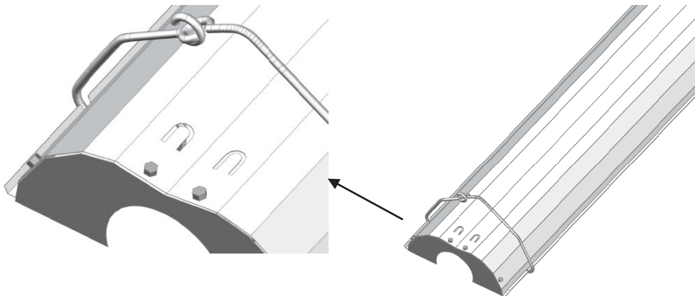
10.ábra: Kombinált tartó felhelyezés
