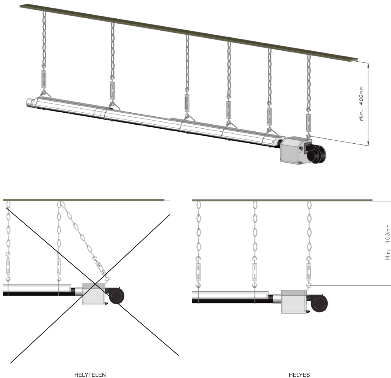
22.ábra: Felfüggesztési megoldások
