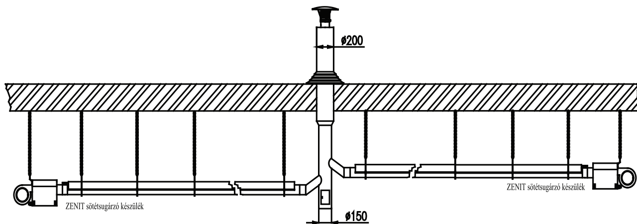
28. ábra: Füstcsatorna kivezetés közös csőben
