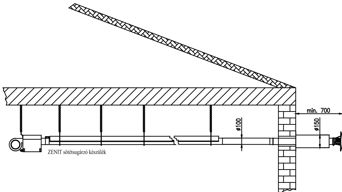
25. ábra: Füstcsatorna kivezetése oldalfalon
